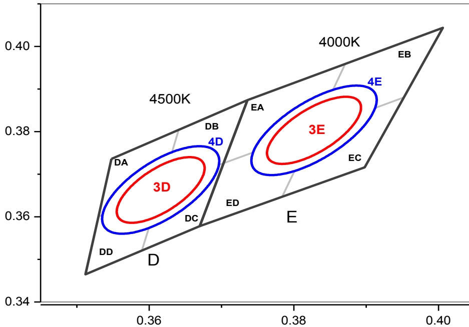
4500K 3Step
